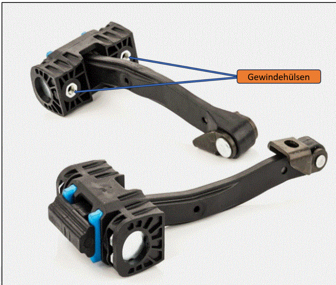
Bild 1: Werkstattbild: Türfeststeller Porsche Macan Neuteile
